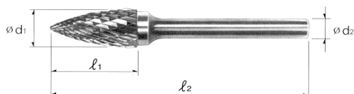
Dubbele vertanding
